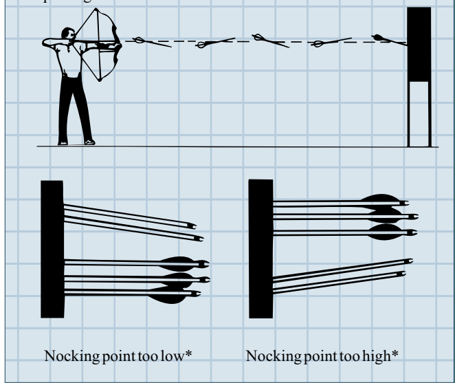
Fig. 10 Porpoising
